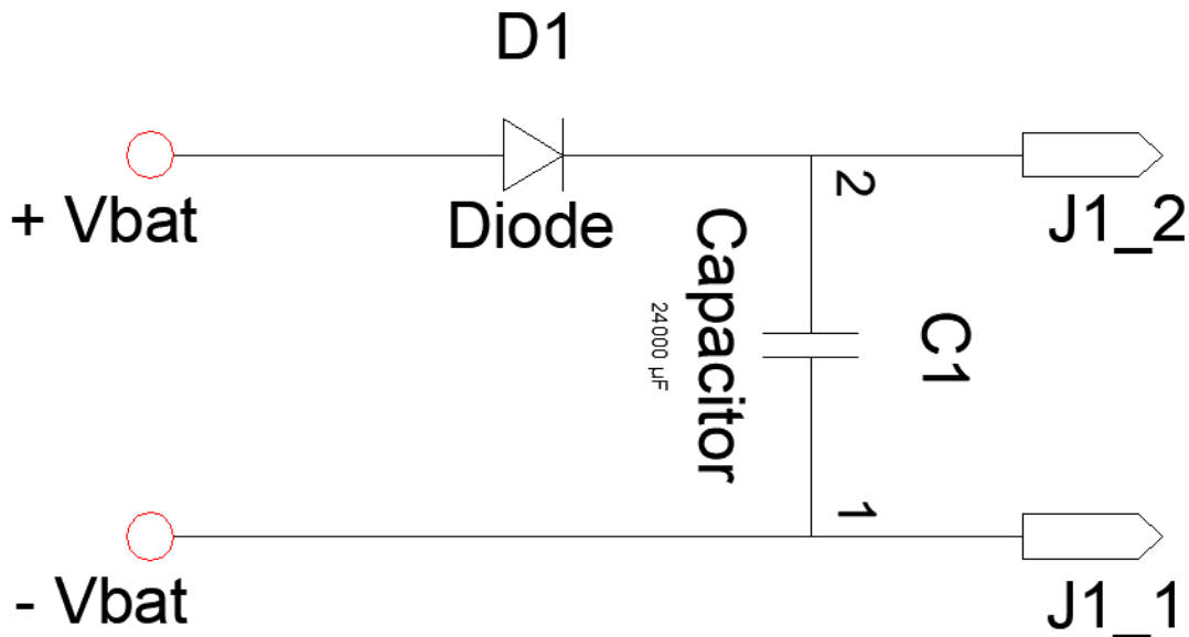
Figure 9. Câblage de l'alimentation 12VDC
