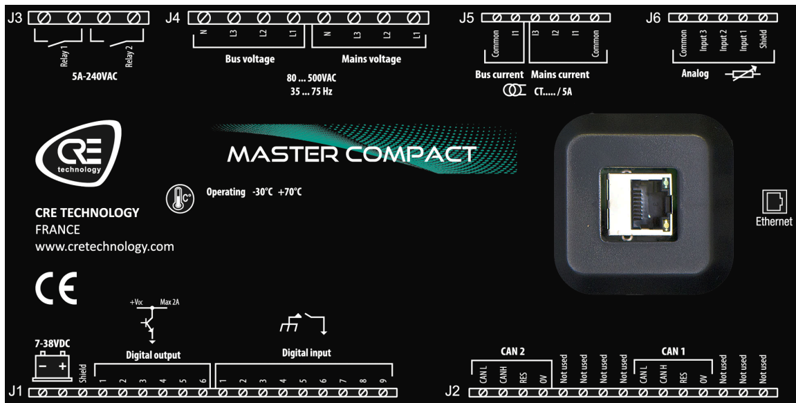
Figure 2. Face arrière d'un contrôleur MASTER COMPACT 1B
