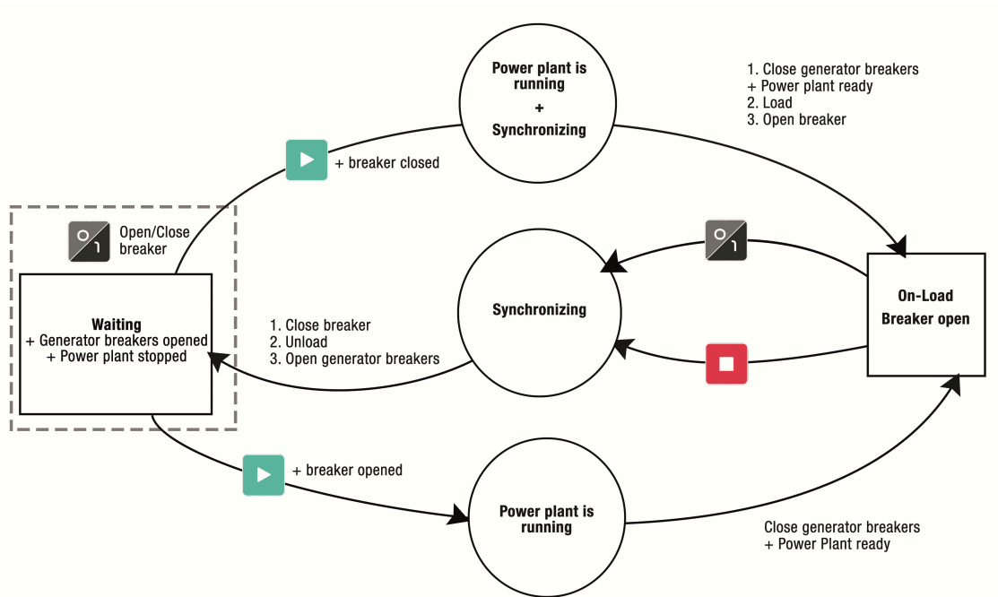
Figure 33. Fugitif: schéma du mode de fonctionnement
