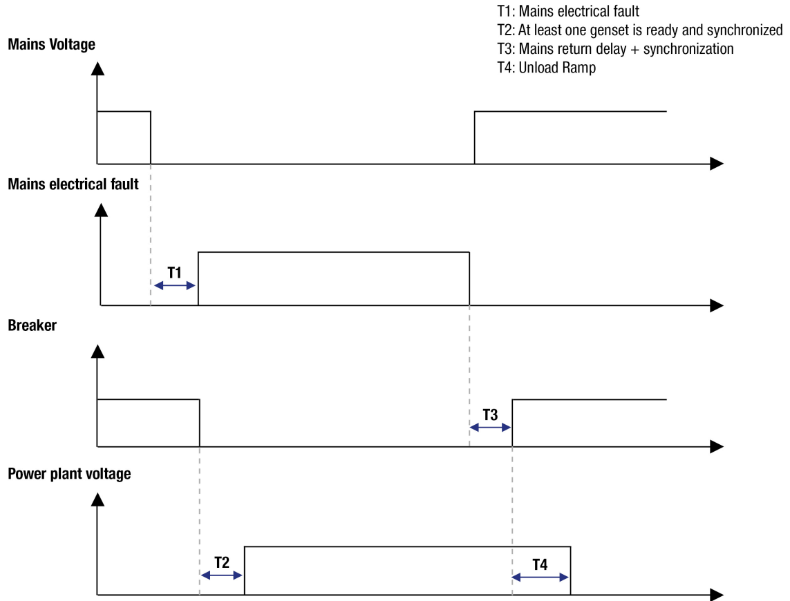
Figure 32. Fugitif lorsque le démarrage distant est désactivé
