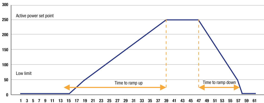
Figure 22. Chronogramme de la rampe de lestage/délestage
