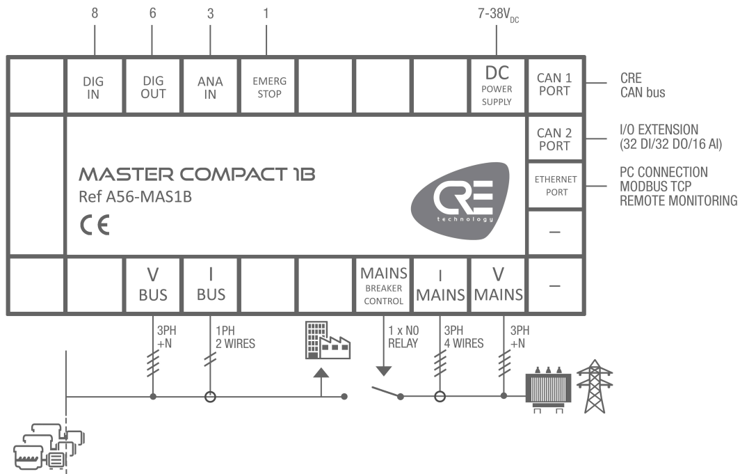
Figure 3. Schéma de câblage simplifié
