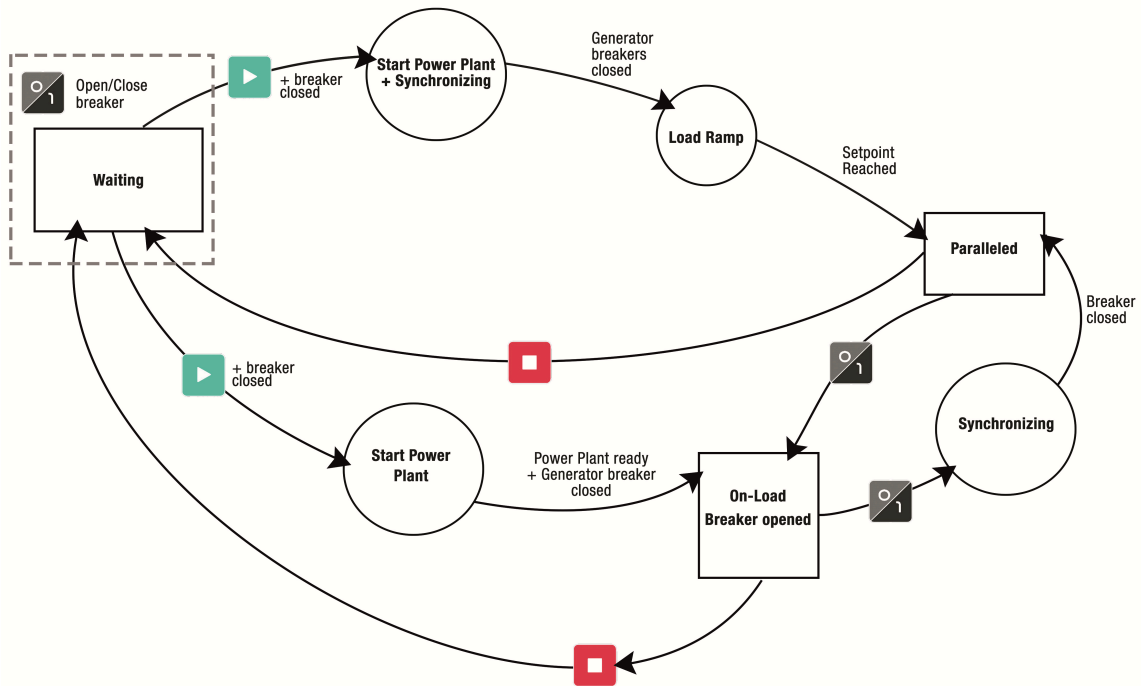
Figure 35. Permanent : schéma du mode de fonctionnement
