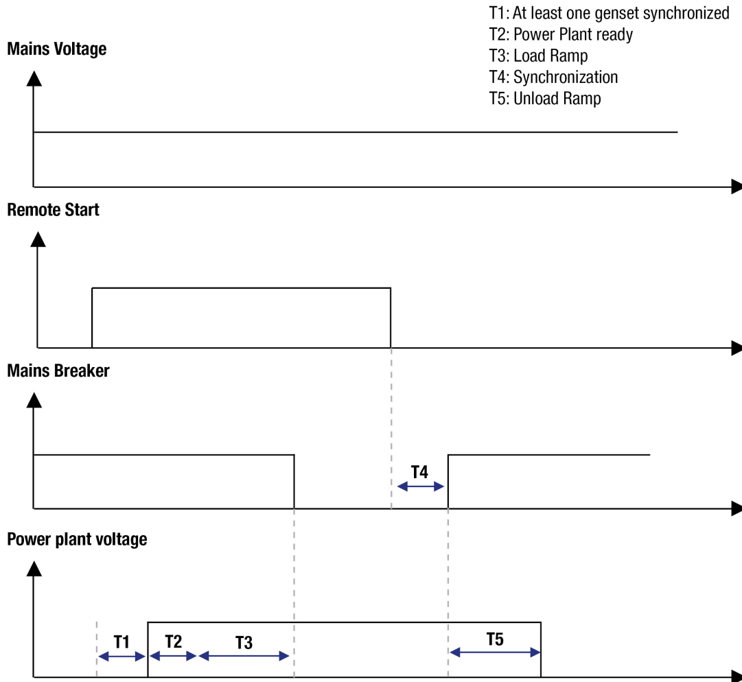
Figure 31. Fugitif avec démarrage distant
