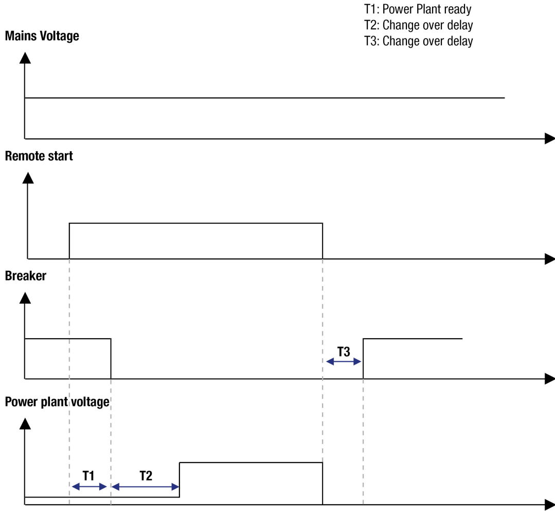
Figure 29. Mode normal/secours avec démarrage distant
