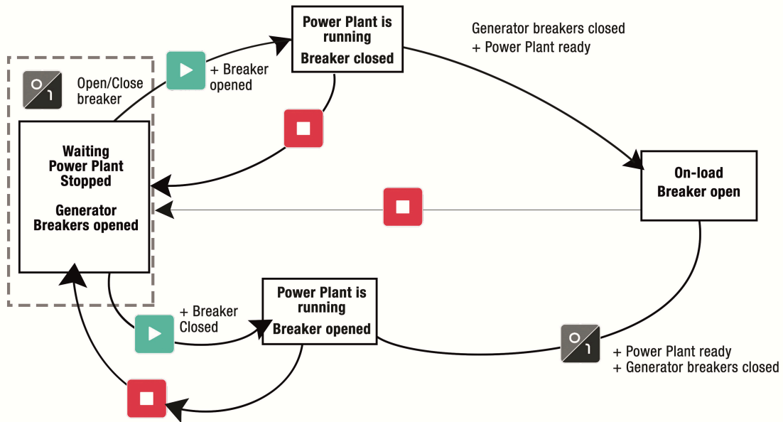
Figure 30. Normal/secours: schéma du mode de fonctionnement
