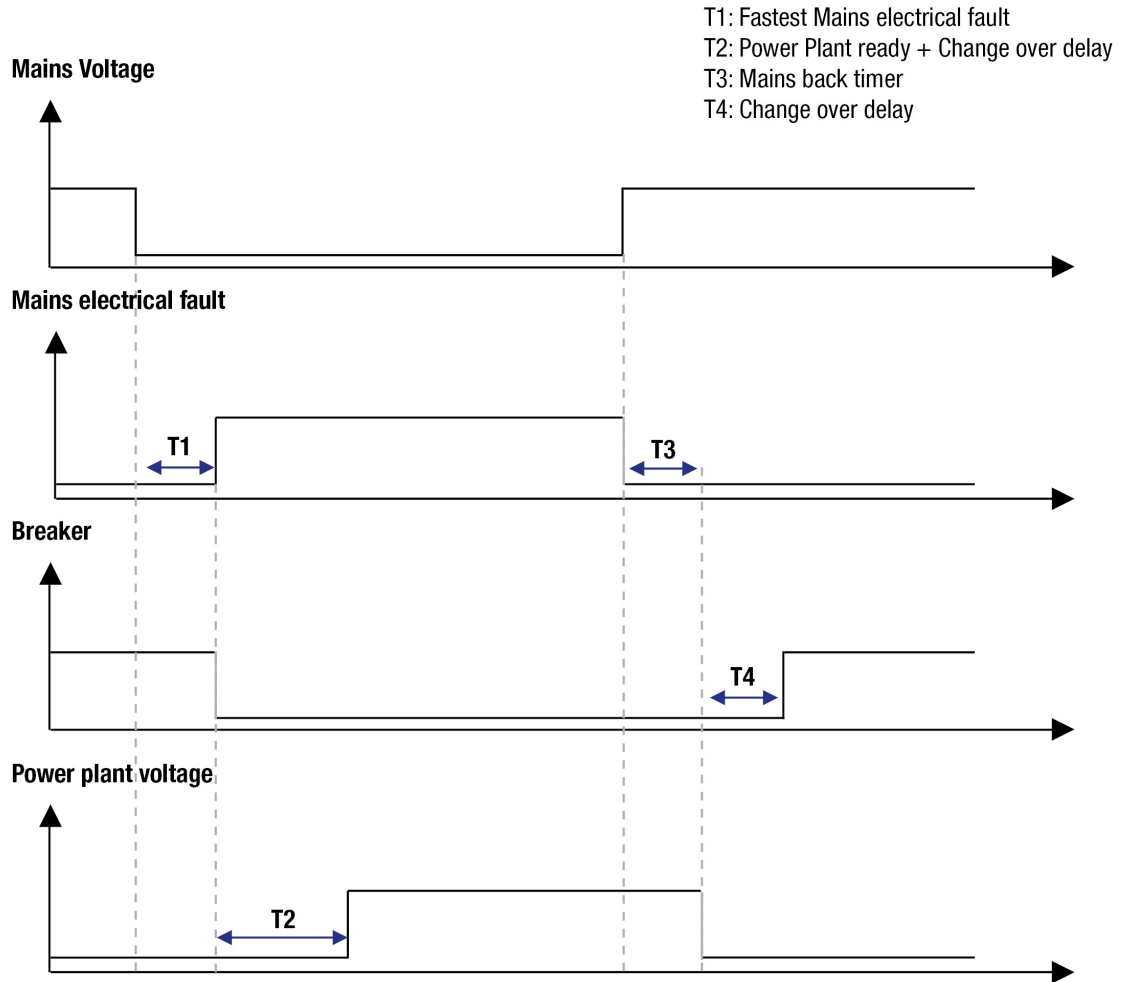
Figure 28. Mode normal/secours en cas de perte secteur
