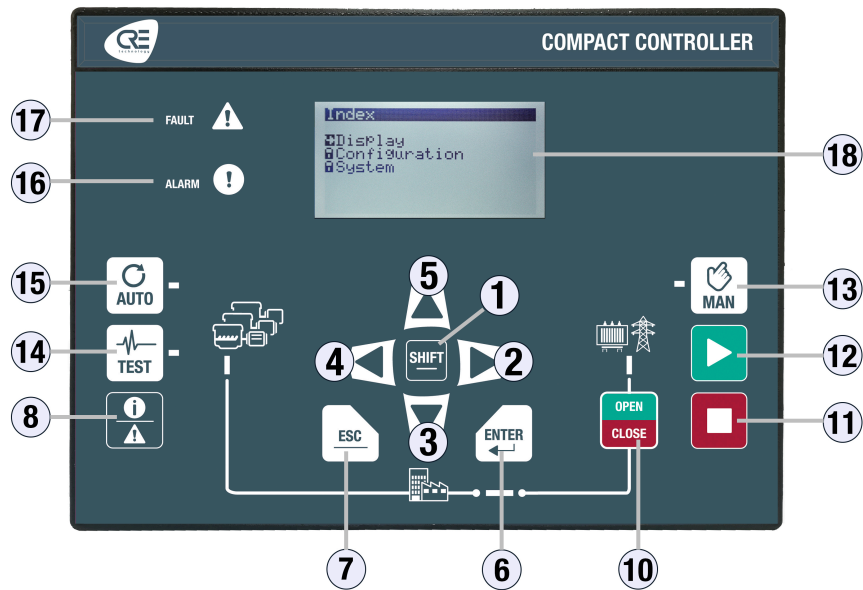
Figure 1. Face avant d'un contrôleur MASTER COMPACT 1B
