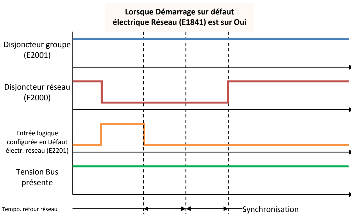
FIGURE 57 - COUPLAGE AU RÉSEAU AVEC UNE ENTRÉE LOGIQUE CONFIGURÉE EN "DÉFAUT ÉLECTRIQUE RÉSEAU"
