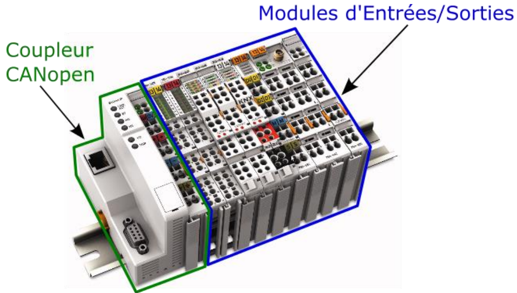
FIGURE 88 - MODULES D'EXTENSION D'ENTRÉES/SORTIES CANOPEN
