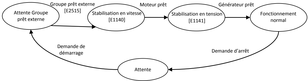
FIGURE 60 - SÉQUENCE DÉMARRAGE EXTERNE
