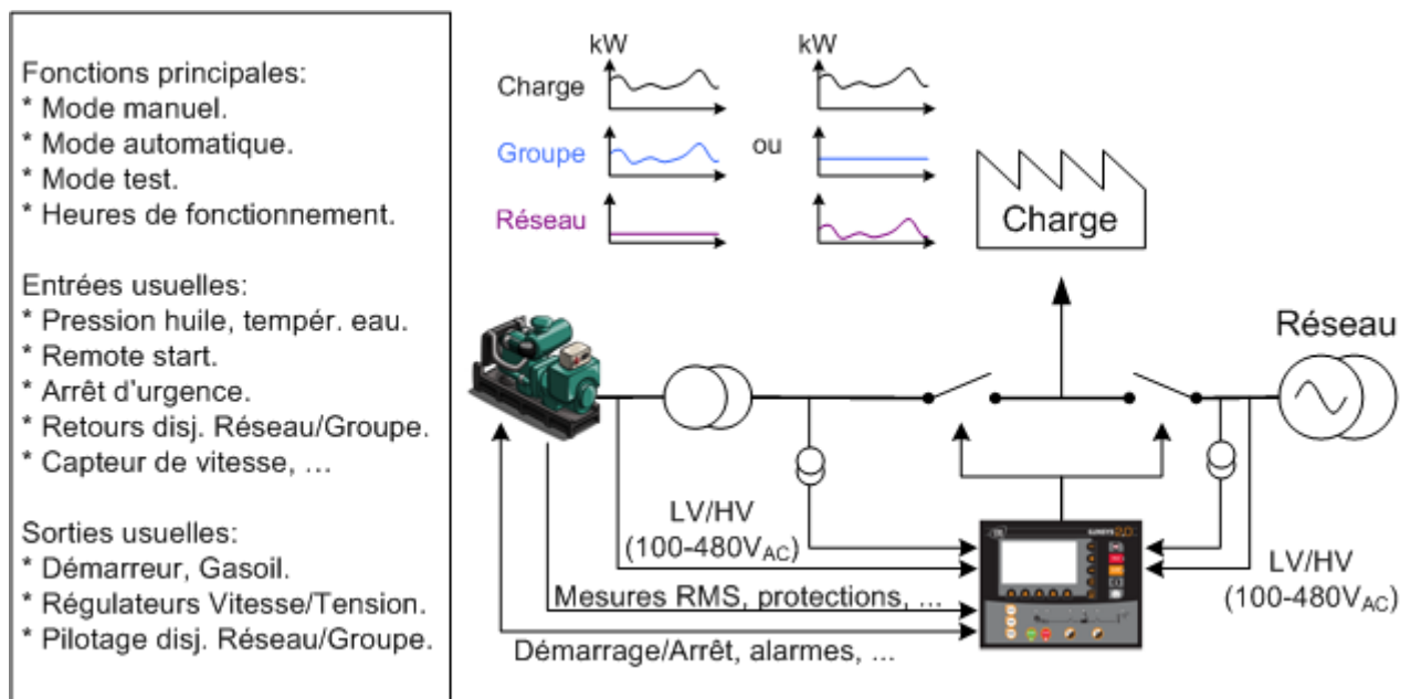
FIGURE 26 - COUPLAGE AU RÉSEAU
