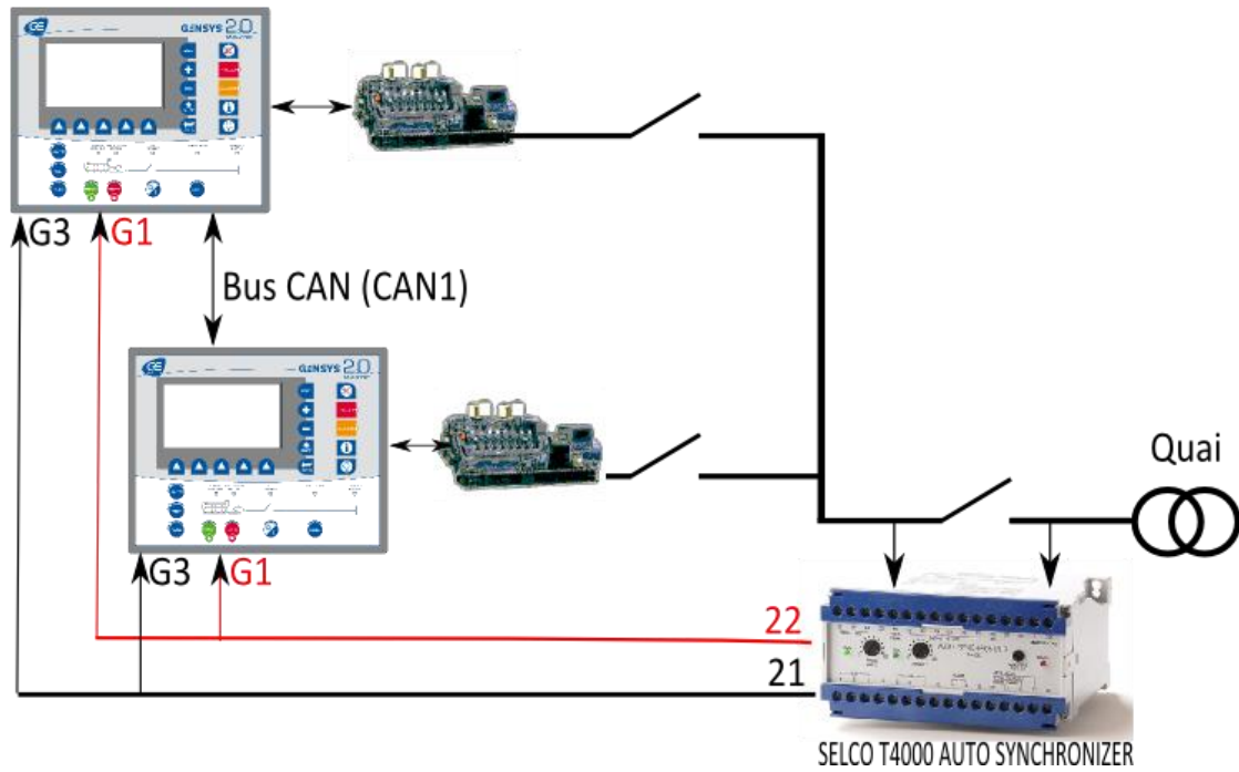
FIGURE 76 - CONNEXION AU QUAÏ À L'AIDE D'UN SELCO T4000
