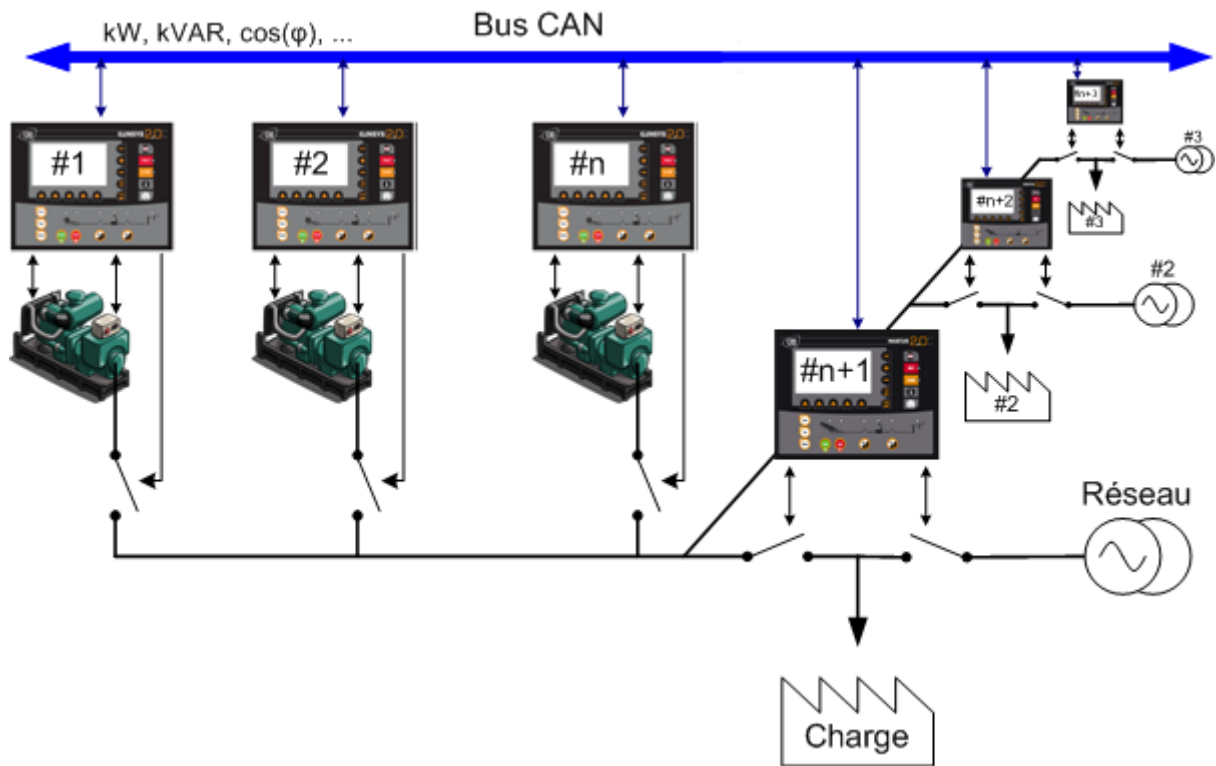
FIGURE 31 - CENTRALE COUPLÉE AVEC PLUSIEURS RÉSEAUX
