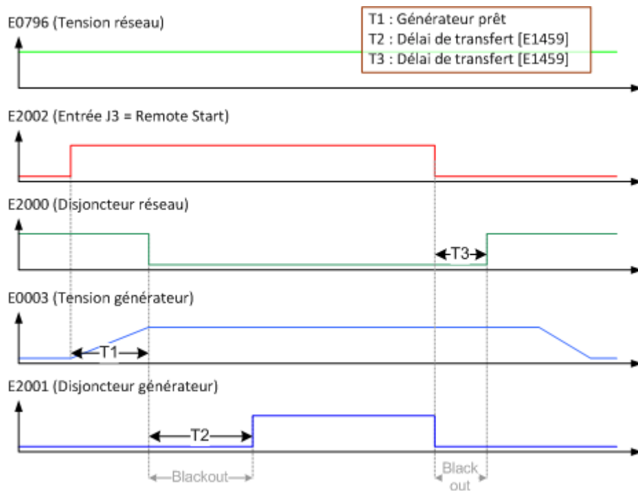
FIGURE 20 - SÉQUENCE TYPE EN MODE NORMAL/SECOURS SUR DEMANDE DE DÉMARRAGE EXTERNE
