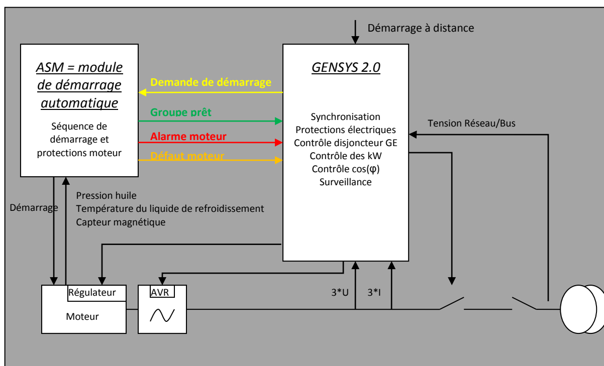
FIGURE 59 - CÂBLAGE ENTRE LE GENSYS 2.0 ET LE MODULE DE DÉMARRAGE AUTOMATIQUE
