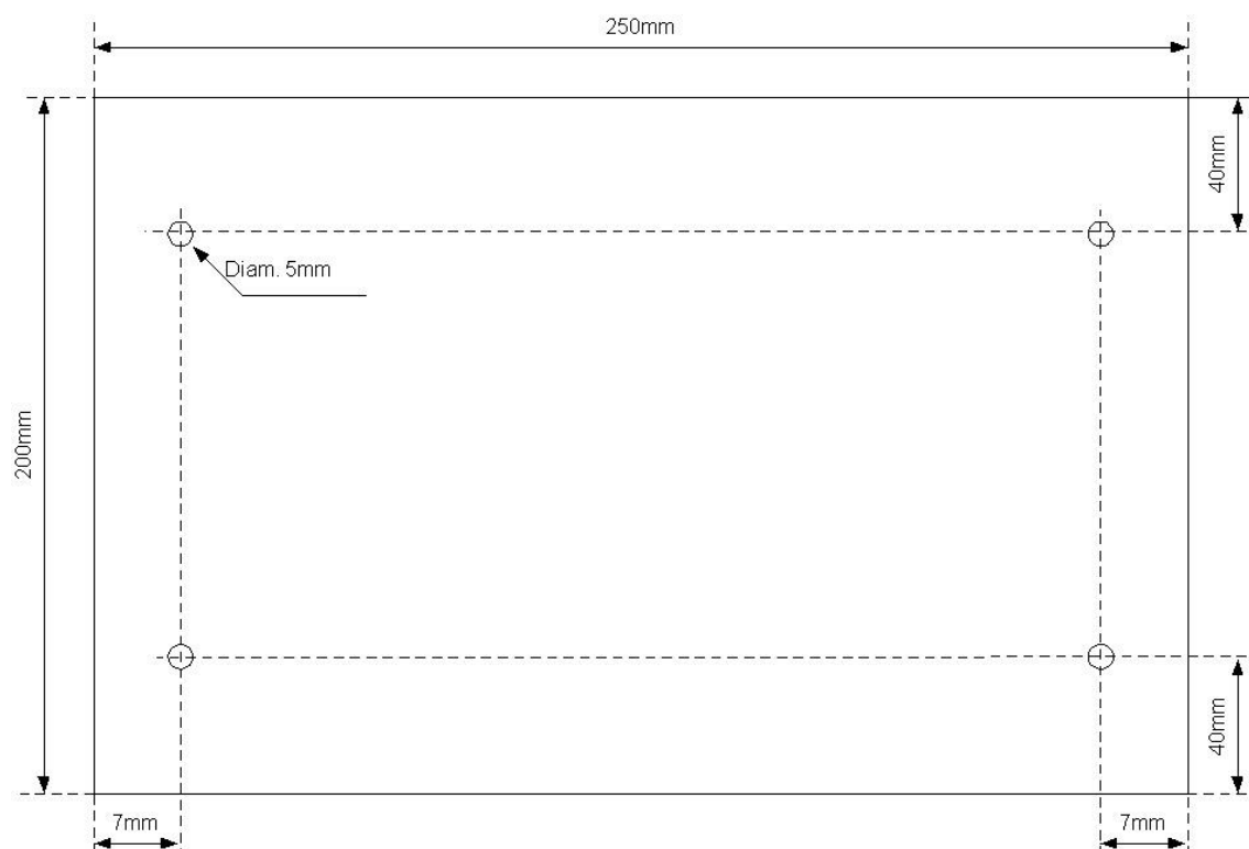
FIGURE 2 - PLAN D'INTÉGRATION DU GENSYS 2.0 CORE
