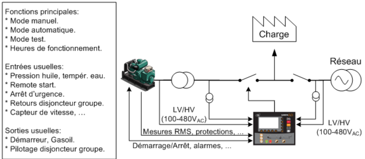
FIGURE 21 - UN SEUL GÉNÉRATEUR SANS NORMAL/SECOURS
