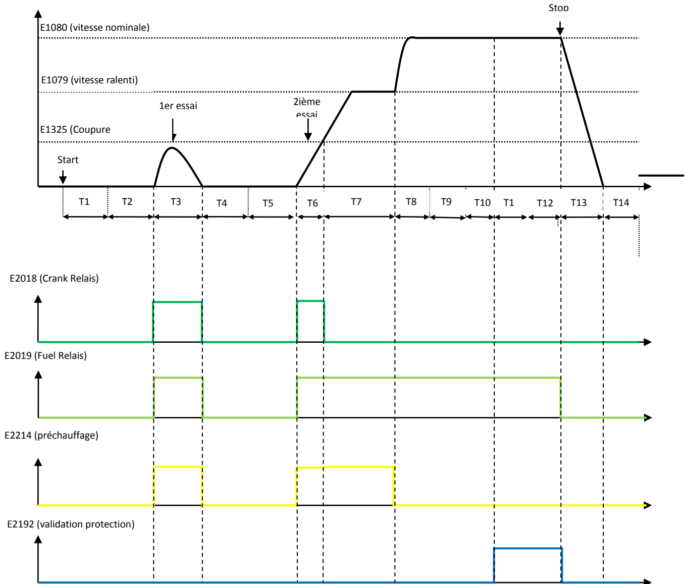
FIGURE 17 - SÉQUENCE DE DÉMARRAGE TYPE
