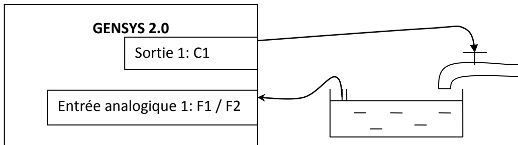
FIGURE 54 - EXEMPLE DE REMPLISSAGE
