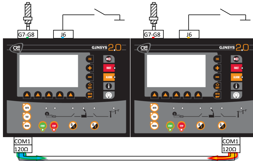
FIGURE 86 - EXEMPLE ÉCHANGE DE DONNÉES PAR BUS CAN
