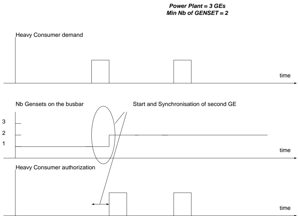
FIGURE 71 - CONTRÔLE DE GROS CONSOMMATEUR AVEC ANALYSE DU NOMBRE DE GROUPES
