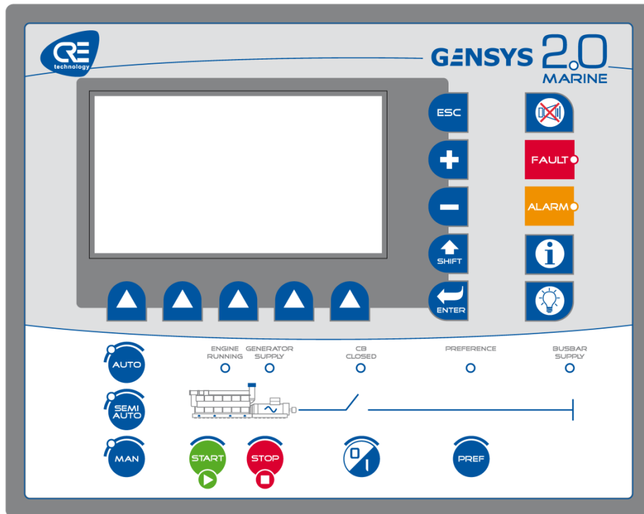
FIGURE 4 - FACE AVANT GENSYS 2.0 MARINE
