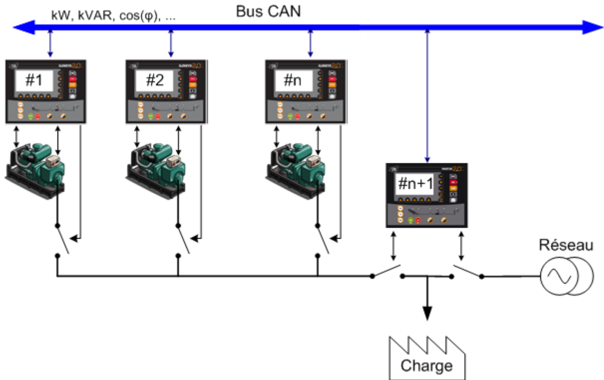
FIGURE 29 - USINE COUPLÉE AU RÉSEAU
