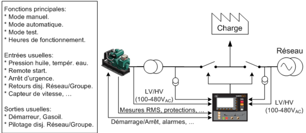
FIGURE 18 - GÉNÉRATEUR EN MODE NORMAL/SECOURS SANS COUPLAGE
