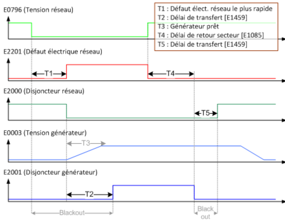
FIGURE 19 - SÉQUENCE TYPE EN MODE NORMAL/SECOURS SUR DÉFAUT ÉLECTRIQUE RÉSEAU
