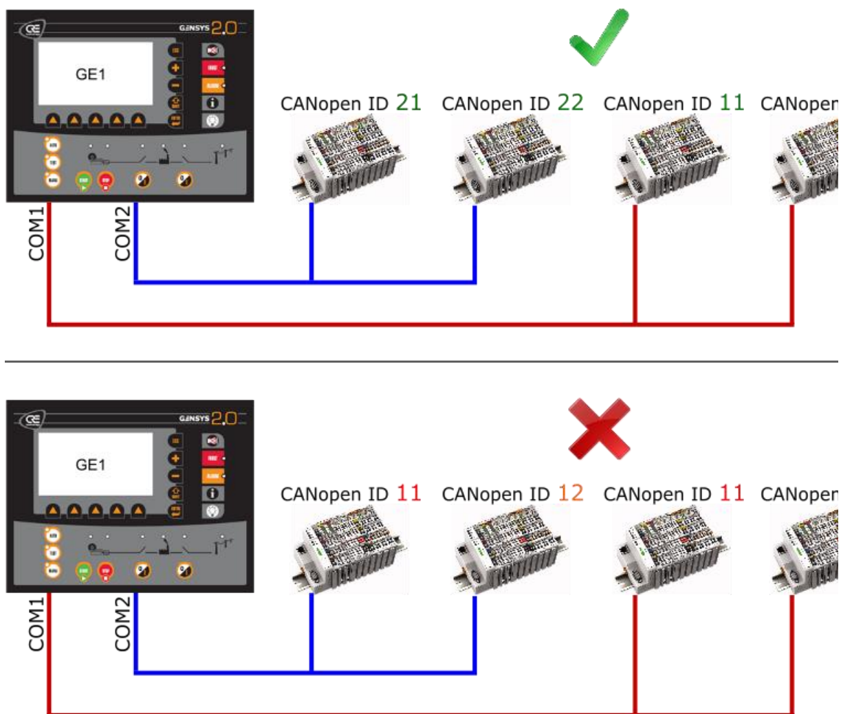
FIGURE 81 - REDONDANCE DE MODULES D'ENTRÉES/SORTIES DÉPORTÉES
