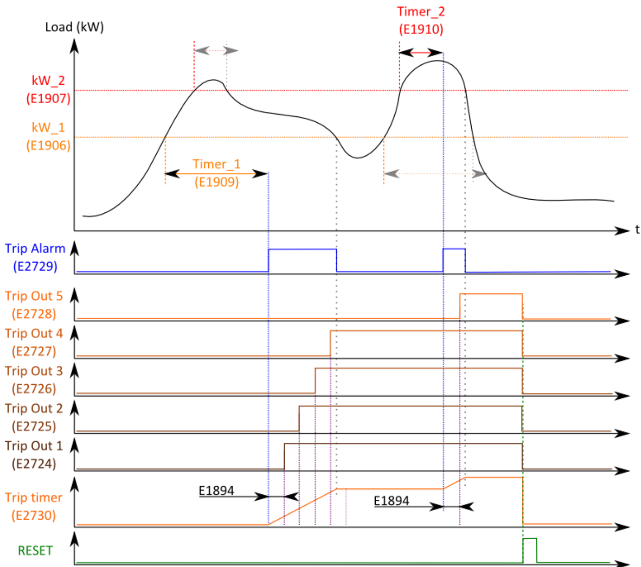
FIGURE 74 - GESTION DES CHARGES NON ESSENTIELLES (KW)
