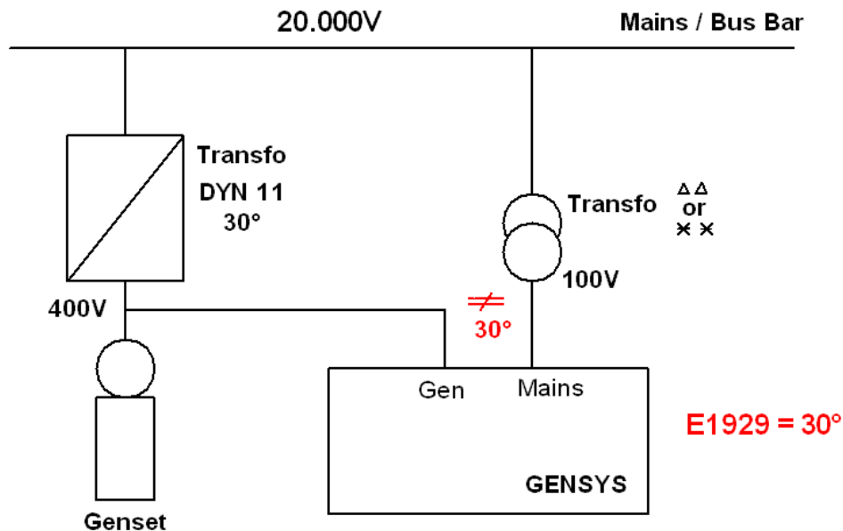
FIGURE 67 - EXEMPLE DE RECALAGE ANGULAIRE
