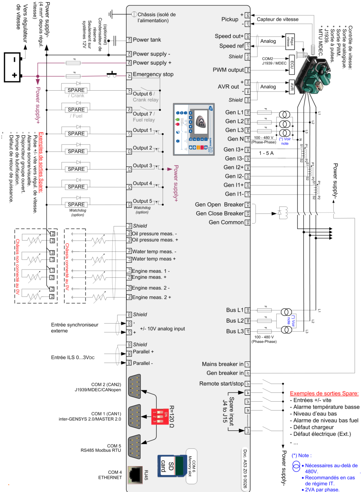
FIGURE 69: CÂBLAGE TYPIQUE (MARINE)
