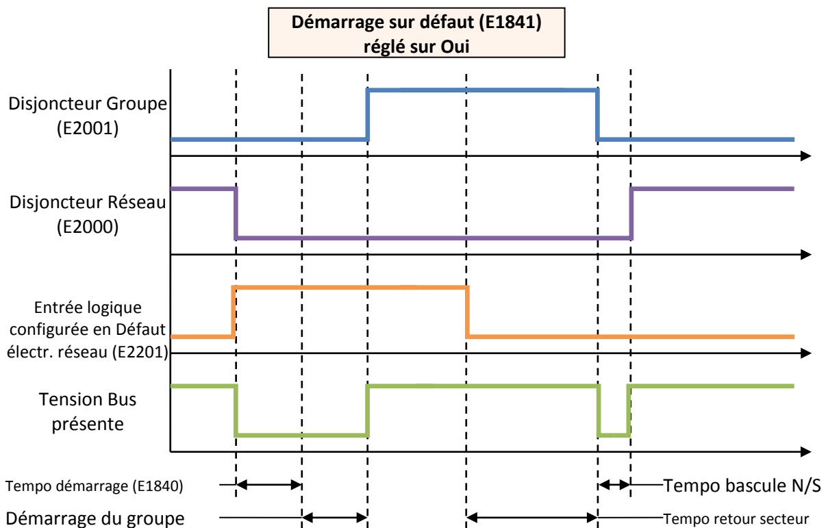
FIGURE 56 - NORMAL/SECOURS AVEC UNE ENTRÉE LOGIQUE CONFIGURÉE EN "DÉFAUT ÉLECTRIQUE RÉSEAU"
