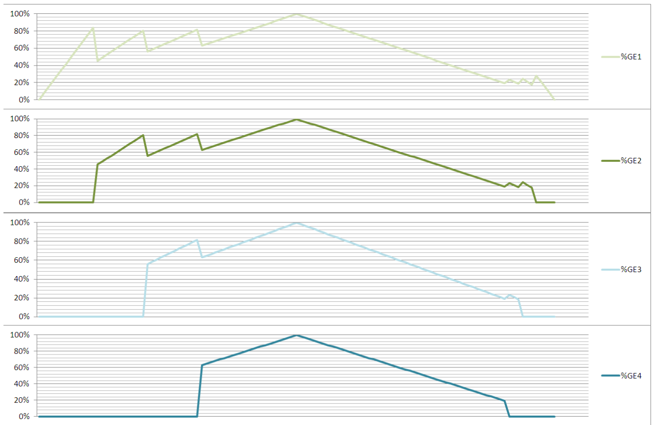
FIGURE 63 - MODE STANDARD - EXEMPLE POUR UNE CENTRALE DE 4X100KW
