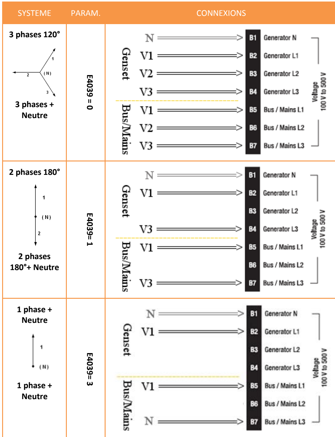
FIGURE 68 - SYSTÈME DE TENSION
