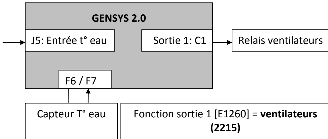
FIGURE 51 - CONNEXION DES VENTILATEURS
