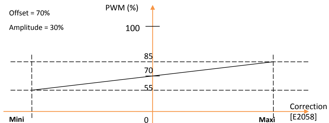
FIGURE 41 - DYNAMIQUE PWM
