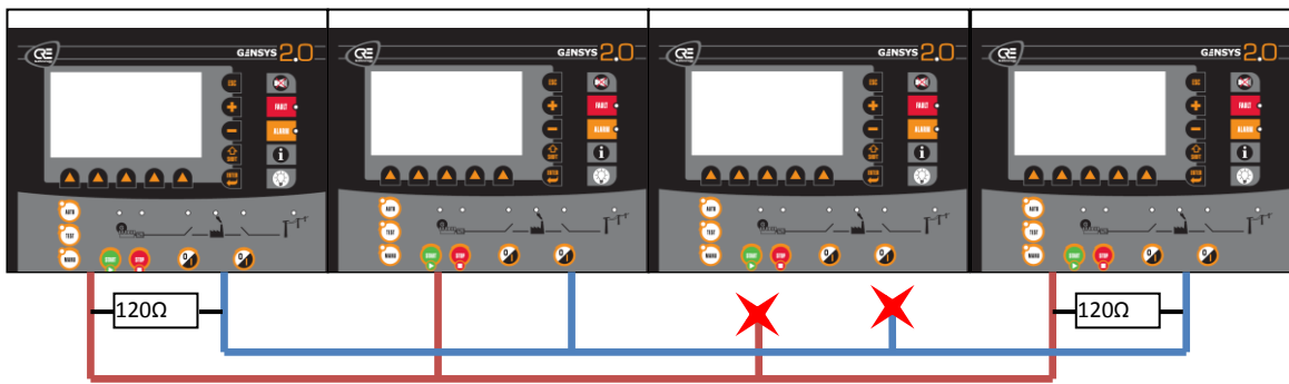
FIGURE 84 - EXEMPLE DÉFAUT BUS CAN
