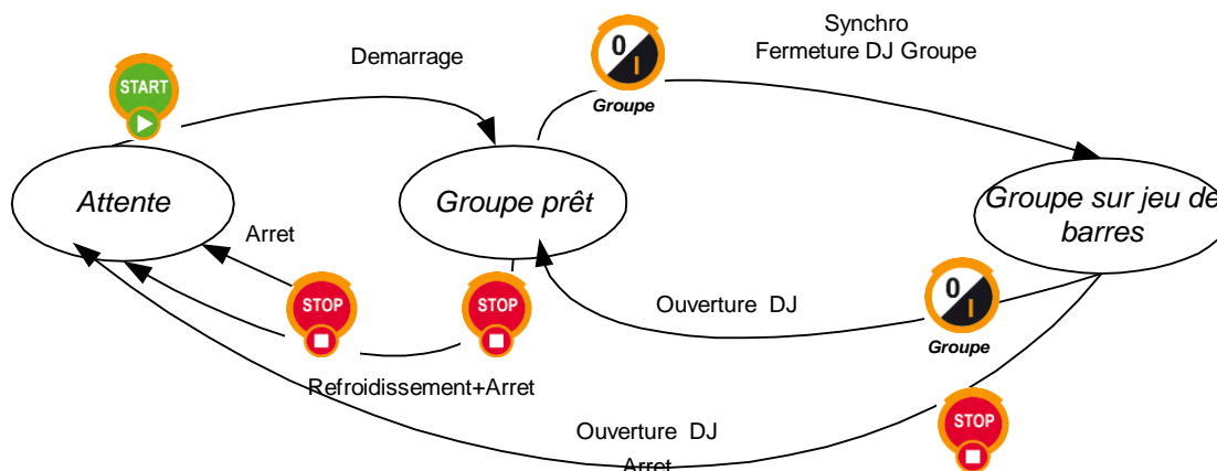
FIGURE 15 - MODE MANUEL ASSISTÉ SANS COUPLAGE RÉSEAU
