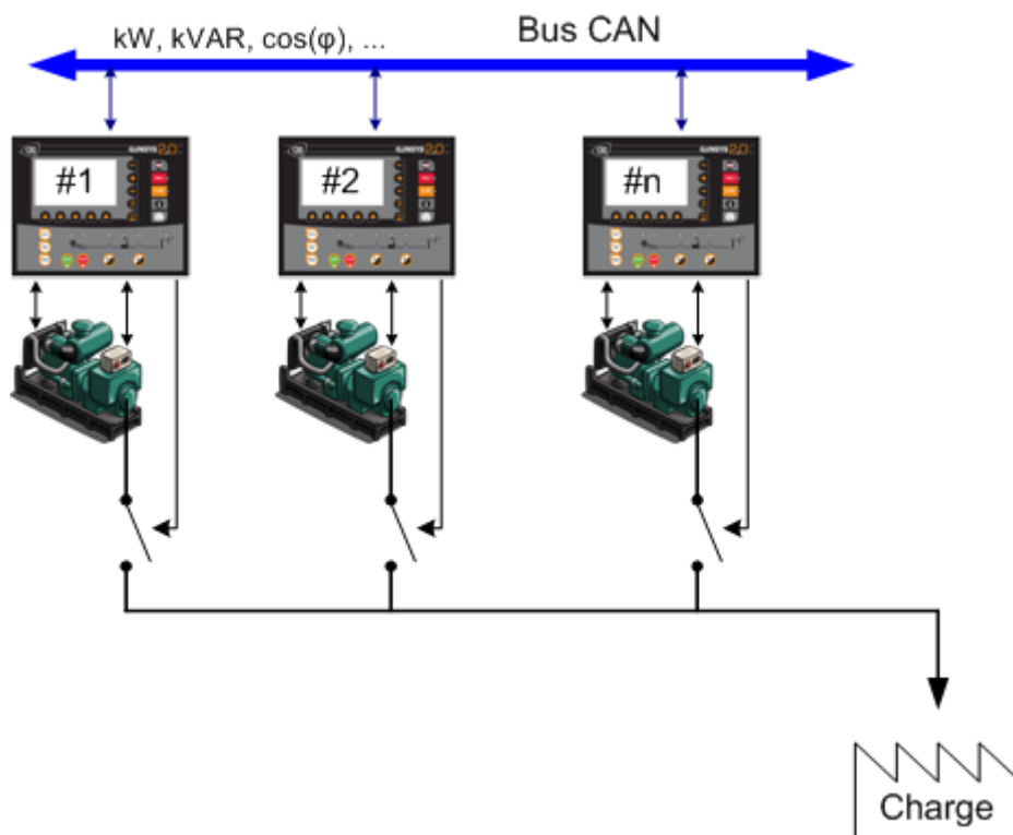
FIGURE 22 - CENTRALE AVEC PLUSIEURS GÉNÉRATEURS
