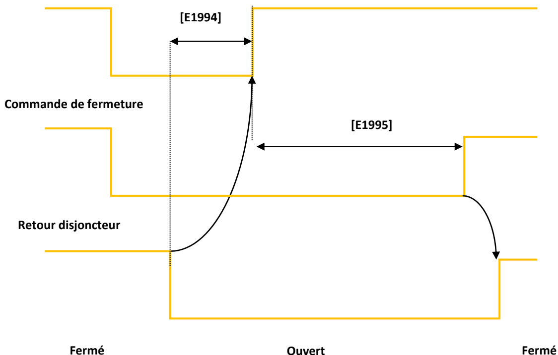
FIGURE 49 - BOBINE À MANQUE
