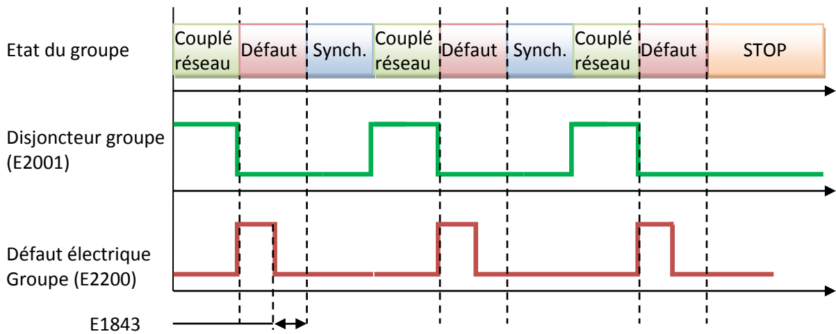
FIGURE 58 - COUPLAGE AU RÉSEAU PERMANENT ET DÉFAUT ÉLECTRIQUE GÉNÉRATEUR
