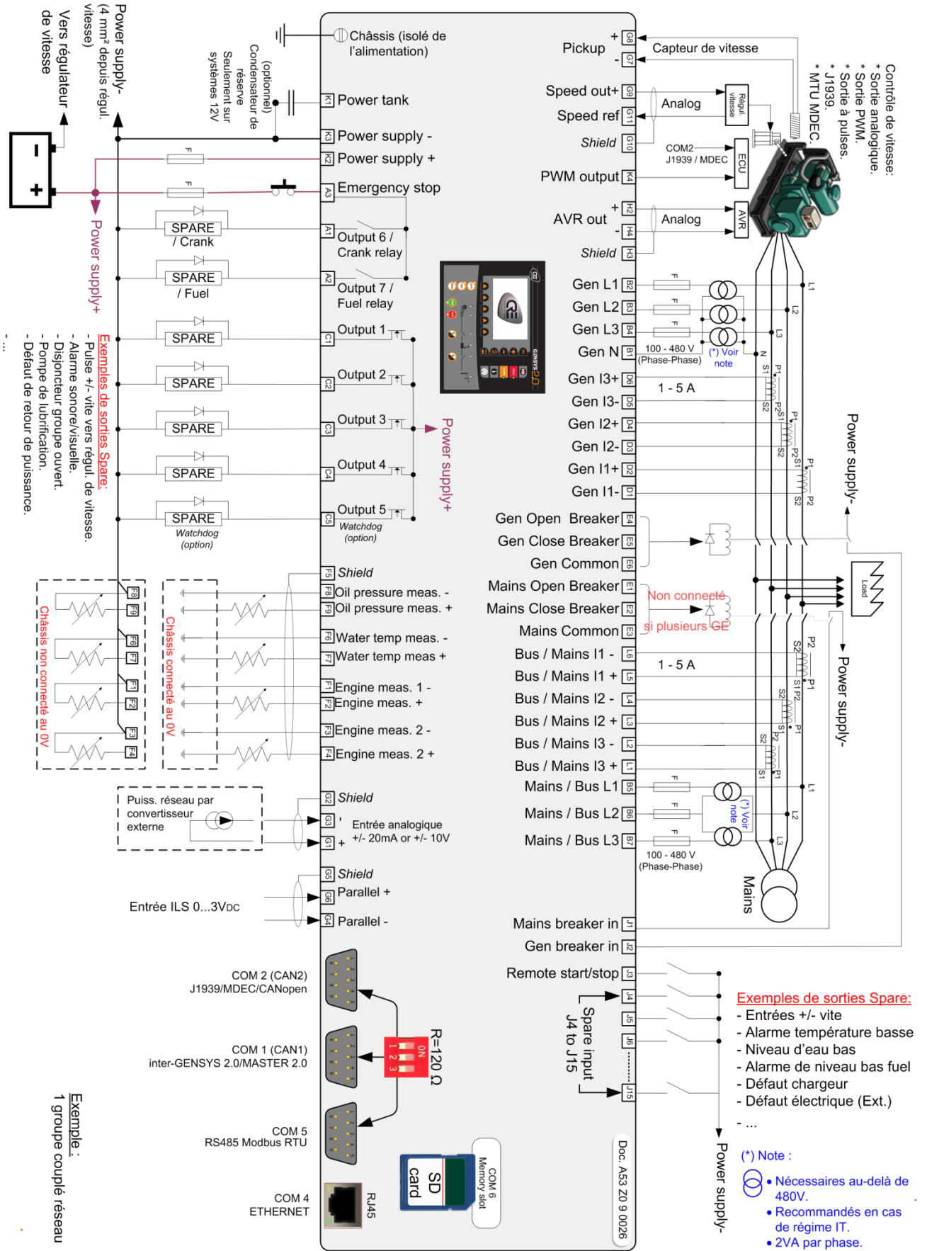
FIGURE 33 - SCHEMA DE CÂBLAGE COMPLET
