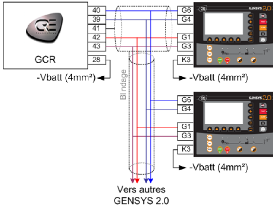
FIGURE 30 - SCHEMA DE CONNEXION GCR ↔ GENSYS 2.0
