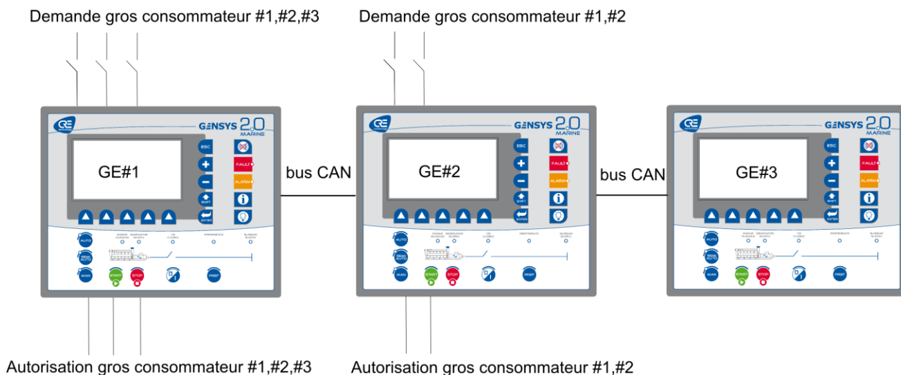
FIGURE 72 - CÂBLAGE TYPIQUE GROS CONSOMMATEUR
