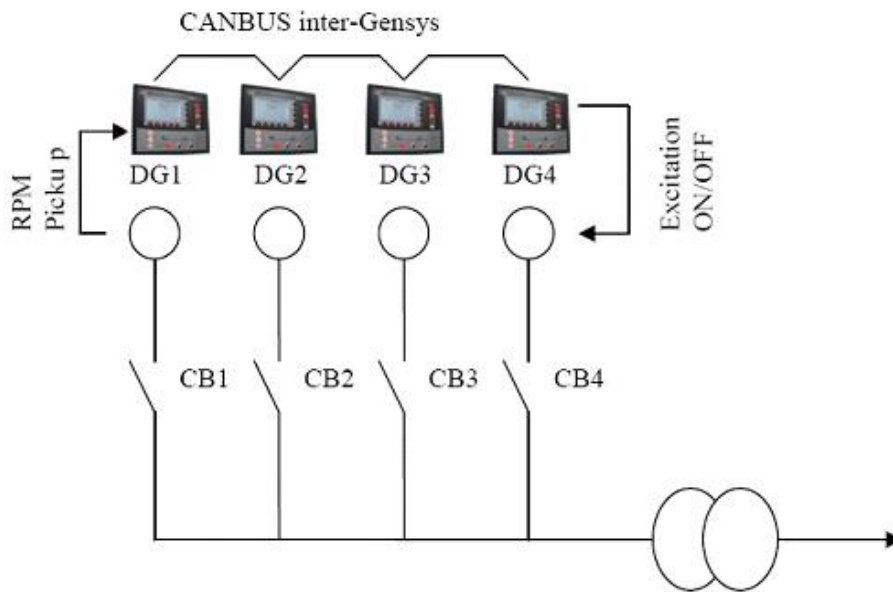
FIGURE 24 - COUPLAGE À L'ARRÊT AVEC 4 GÉNÉRATEURS EN SITUATION D'URGENCE
