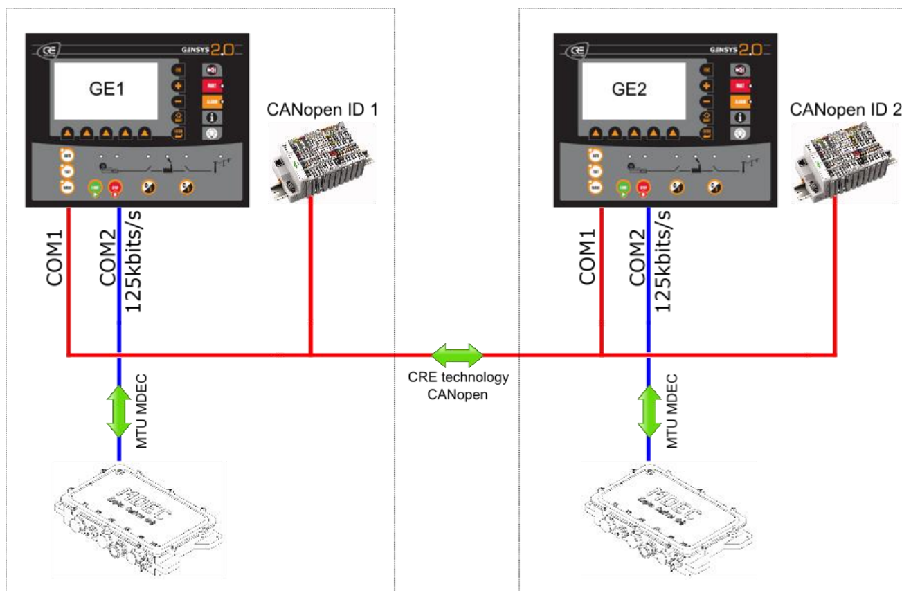
FIGURE 82 - REDONDANCE DE MODULES D'ENTRÉES/SORTIES DÉPORTÉS
