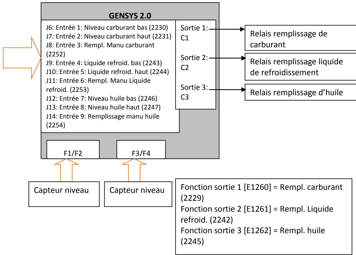
FIGURE 52 - CONNEXIONS POUR LE REMPLISSAGE
