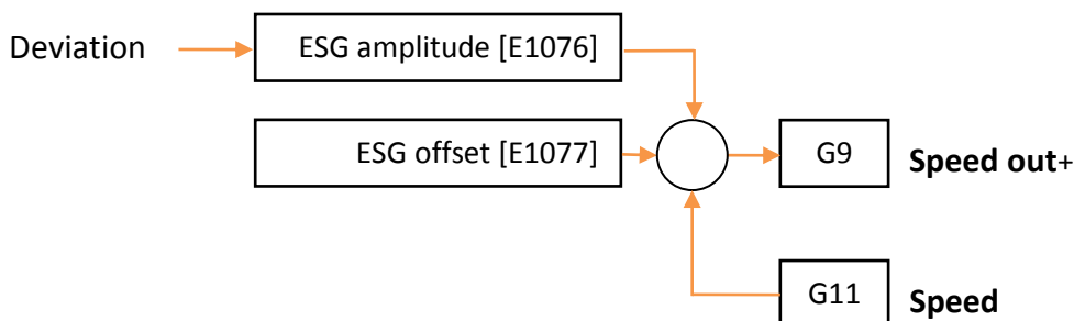
FIGURE 39 - SORTIE VITESSE
