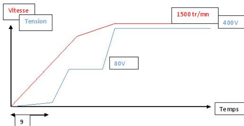
FIGURE 25 - SÉQUENCE DE COUPLAGE À L'ARRÊT AVEC 4 GÉNÉRATEURS EN SITUATION D'URGENCE
