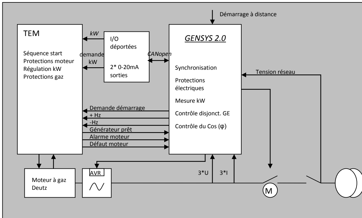
FIGURE 61 - CÂBLAGE GENSYS 2.0 ↔ TEM
