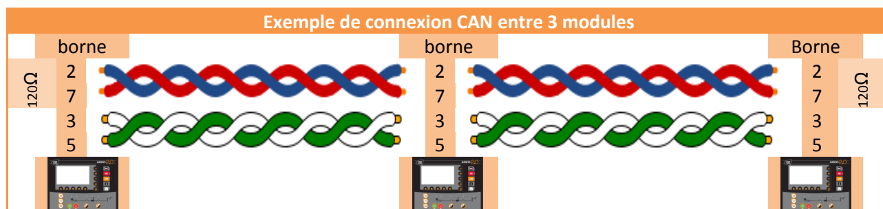
FIGURE 78 - EXEMPLE DE CONNEXION CAN INTER-MODULES
