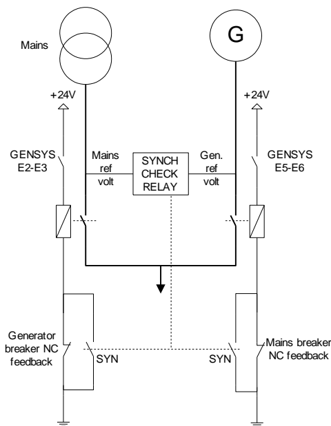
FIGURE 105 - UN GÉNÉRATEUR AVEC LE RÉSEAU
