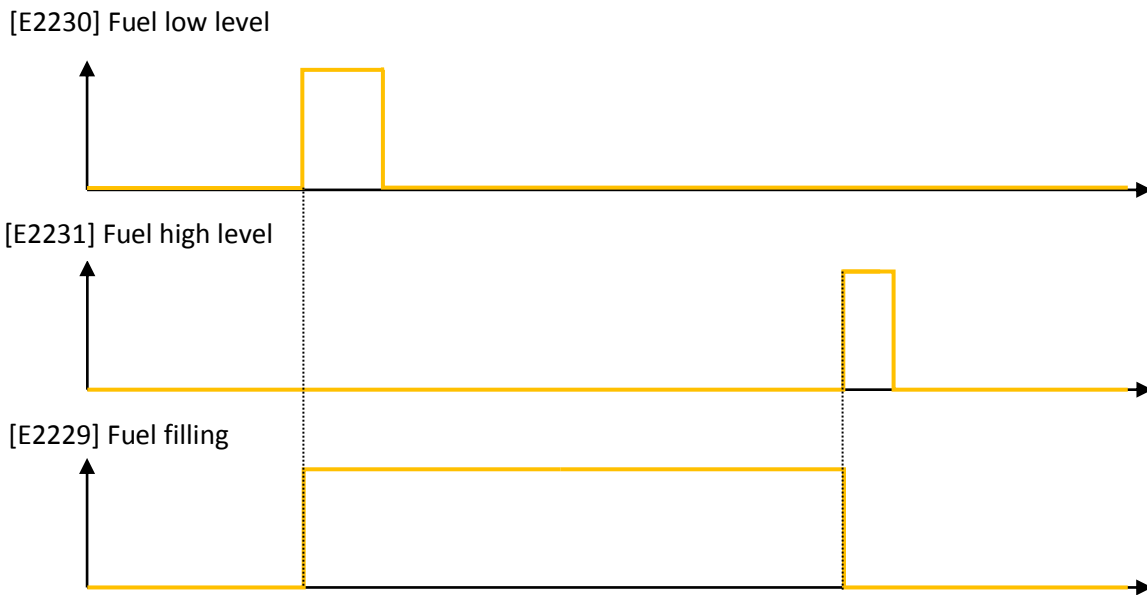
FIGURE 53 - DIAGRAMME DE REMPLISSAGE
