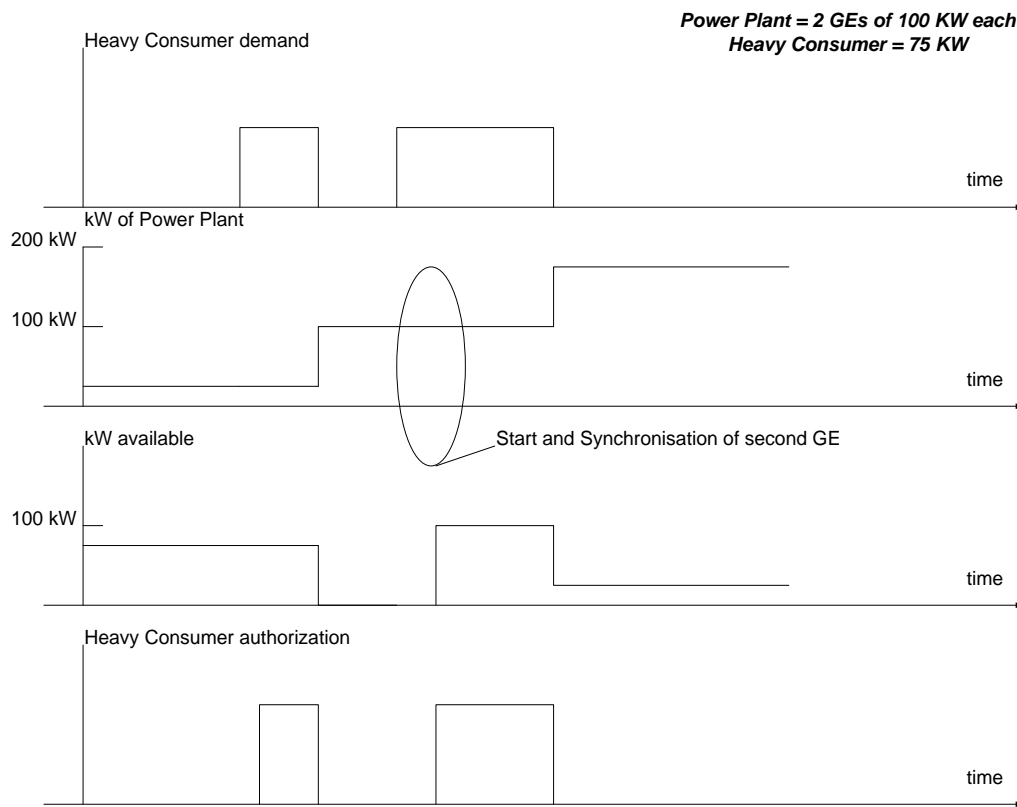
FIGURE 70 - CONTRÔLE DE GROS CONSOMMATEUR AVEC ANALYSE DE LA PUISSANCE ACTIVE
