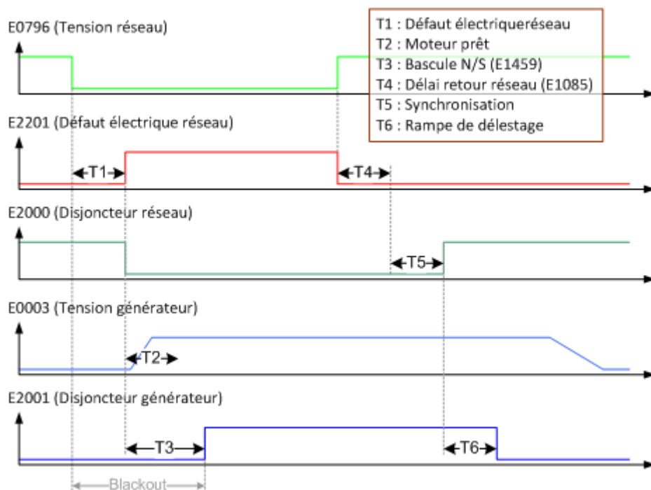
FIGURE 28 - SÉQUENCE TYPE EN MODE FUGITIF SUR DÉFAUT ÉLECTRIQUE RÉSEAU
