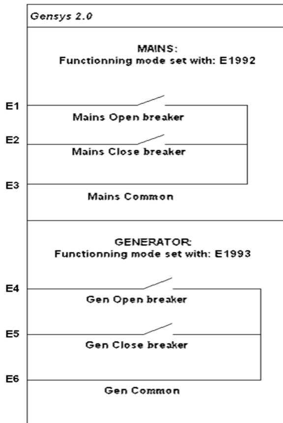
FIGURE 48 - CÂBLAGE DES SORTIES DISJONCTEURS
