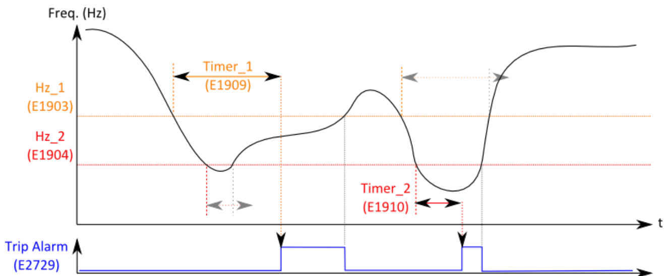
FIGURE 75 - GESTION DES CHARGES NON ESSENTIELLES (HZ)
