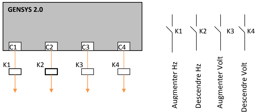
FIGURE 4.3 - RÉGULATEUR DE VITESSE/TENSION PILOTÉ PAR CONTACTS/IMPULSIONS
