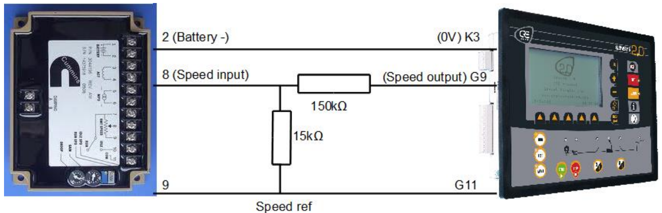
FIGURE 40 - CONNEXION AVEC UN EFC CUMMINS
