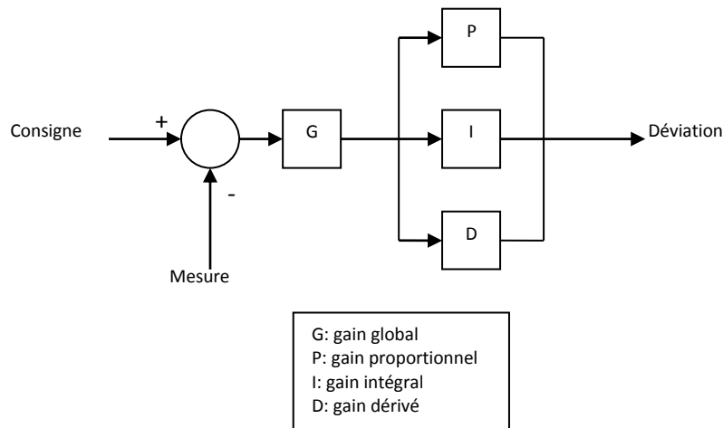
FIGURE 62 - CONTRÔLEUR GPID TYPE
