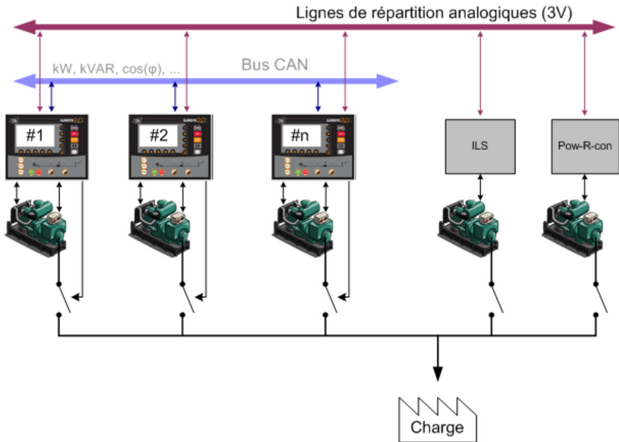
FIGURE 23 - GÉNÉRATEURS COUPLÉS PAR LIGNES PARALLÈLES
