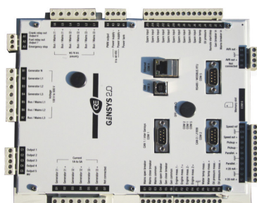
VERSIÓN CORE PARA MONTAJE EN RIEL DIN
