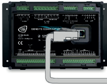
A53W1 (Ethernet) CABLE TRENZADO CAT 5
