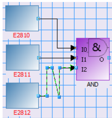
FIGURA 33: CONEXIÓN CON ESQUINAS ADICIONALES
