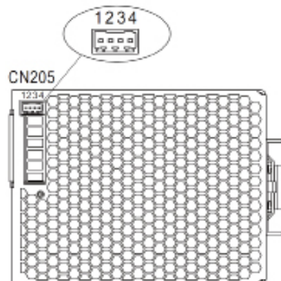
AMMISSIBLE DIN-RAIL: TS35/7.5 OR TS35/15
